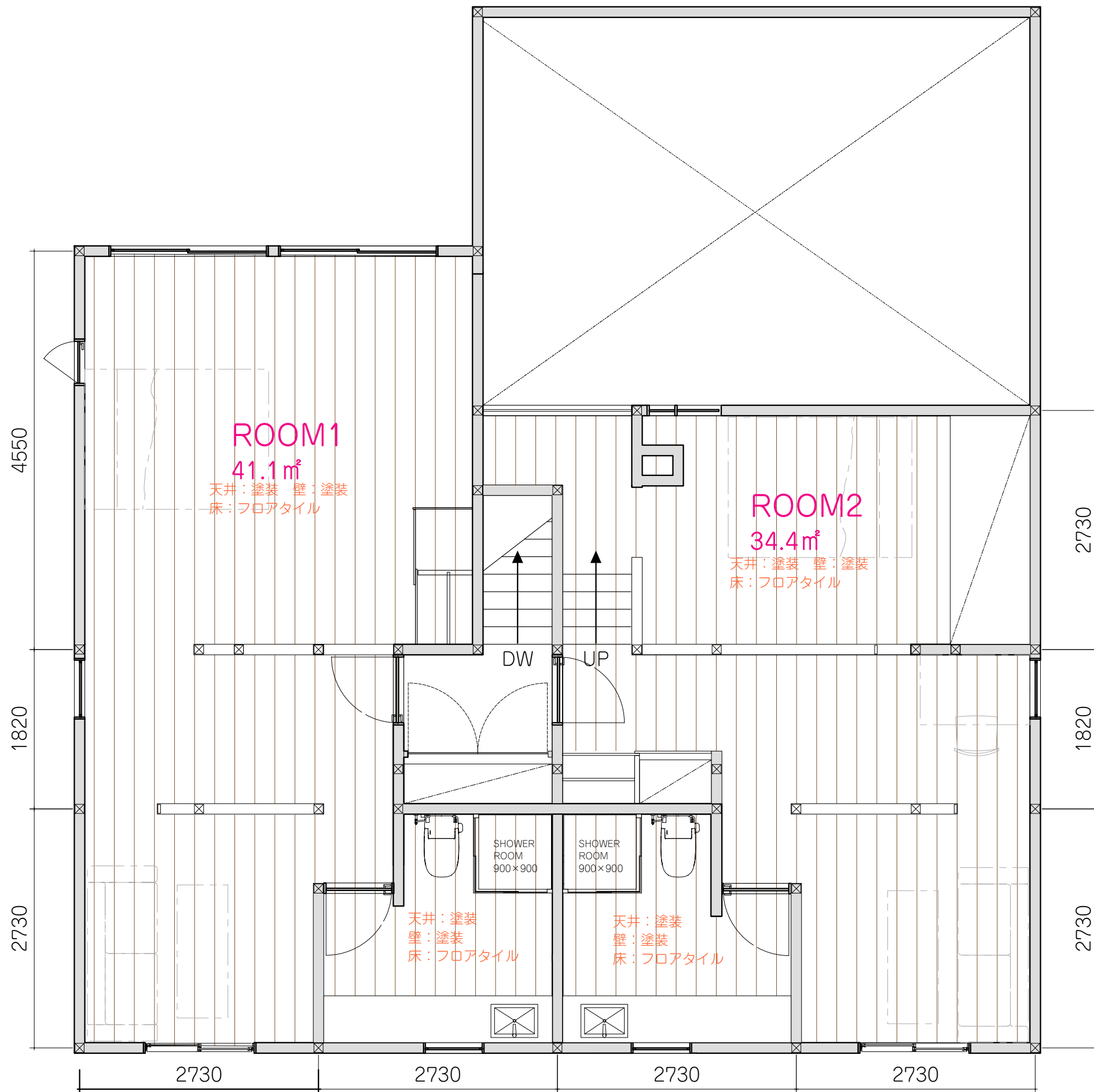
◎2F 平面図 S=50:1
