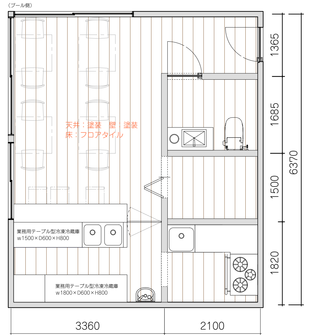
◎別棟 平面図 S=50:1
